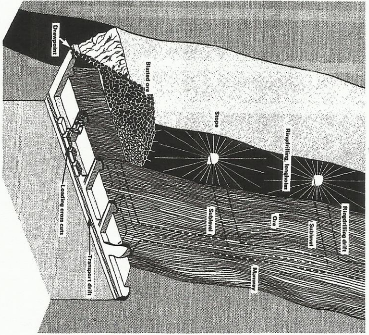
FIGURE 72.9 Sublevel stoping using fan patterns, Atlas Copco (1986)
