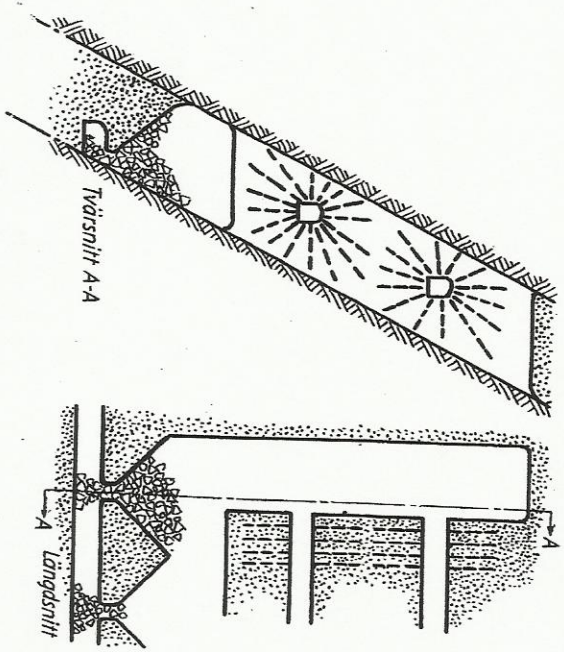
42. Skivpallbrytning med långhål. 100
